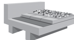
Isolant sur étanchéité RAVATHERM SL (tarif I5)
