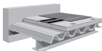
Système par fixation mécanique
